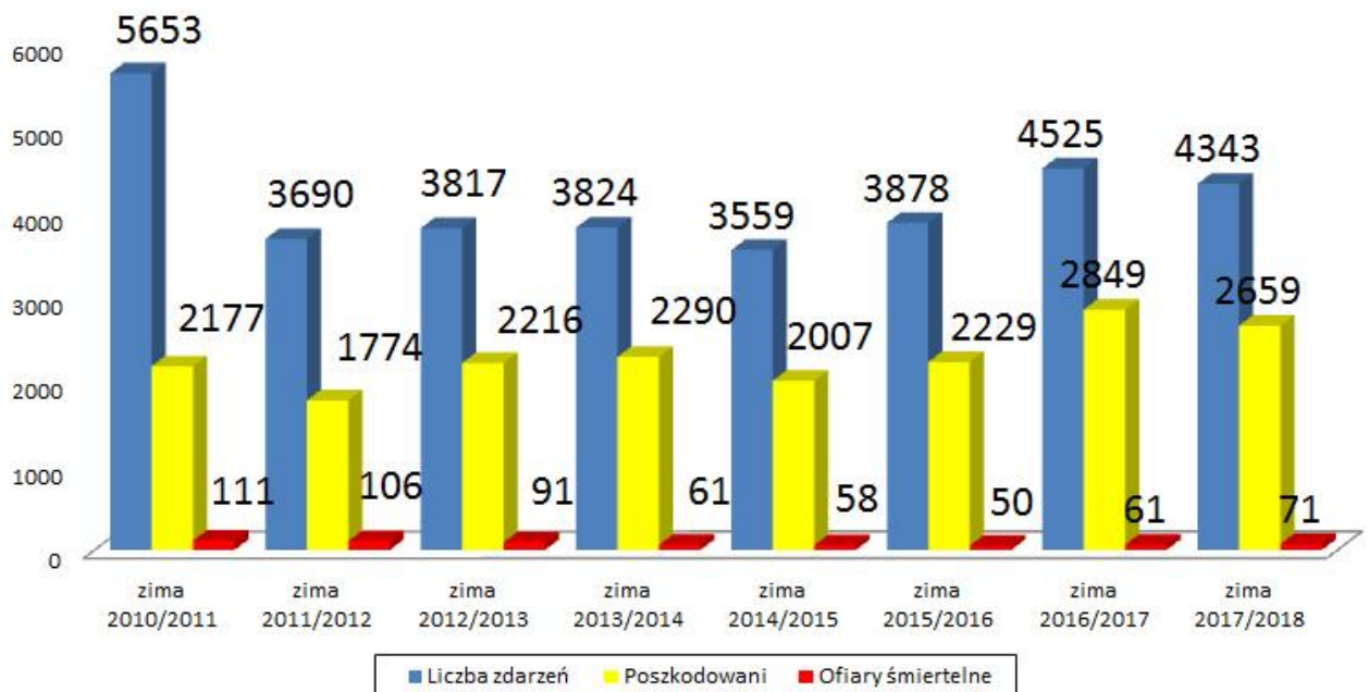
Liczba zdarzeń związanych z tlenkiem węgla, liczba poszkodowanych i ofiar śmiertelnych w sezonach grzewczych 2010/2011, 2011/2012, 2012/2013, 2013/2014, 2014/2015, 2015/2016, 2016/2017, 2017/2018
